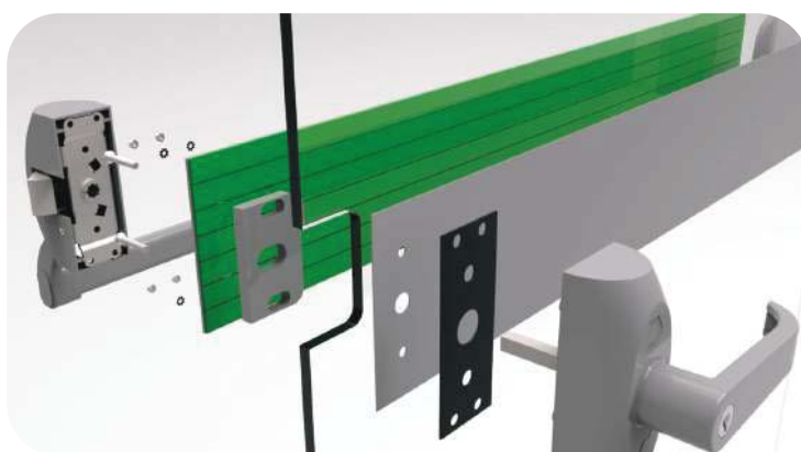
Barra Antipânico Push
