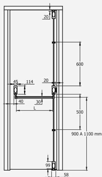
Barra Antipânico Neo 1 Folha com hastes e trincos
