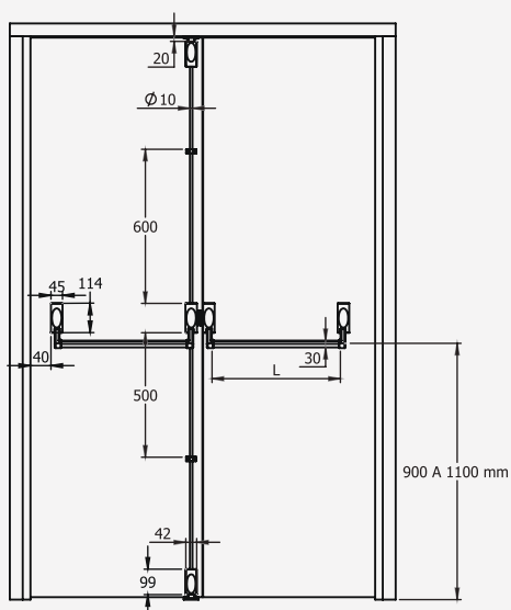
Barra Antipânico Neo 2 Folhas
