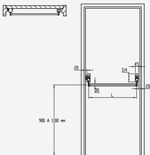
Barra Antipânico Push 1 Folha
