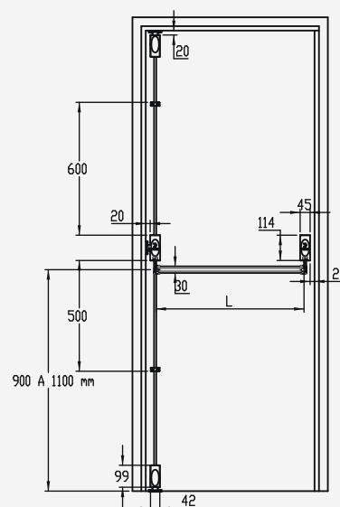
Barra Antipânico Push 1 Folha com hastes e trincos
